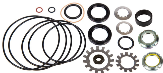
Packningssats underhus/Seal kit lower unit Mutter 814164 ingår ej/Flange nut 814164 is not included
